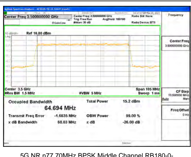
5G NR n77 70MHz BPSK Middle Channel RB180-0
