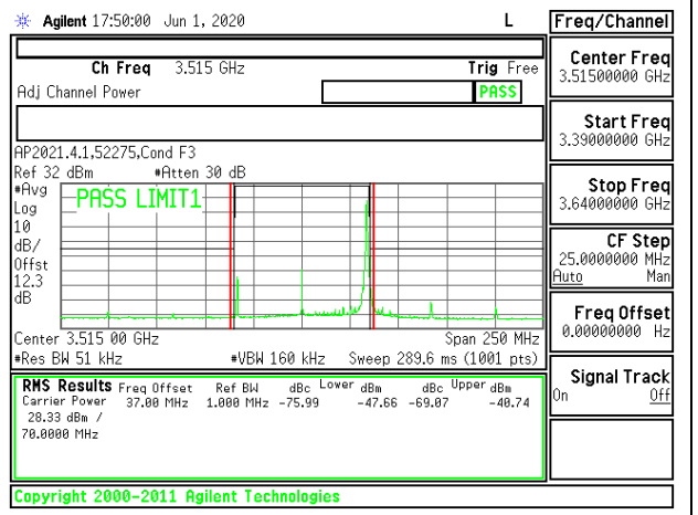
5G NR n77 70MHz BPSK High Channel RB1-187
