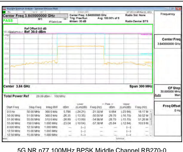
5G NR n77 100MHz BPSK Middle Channel RB270-0
