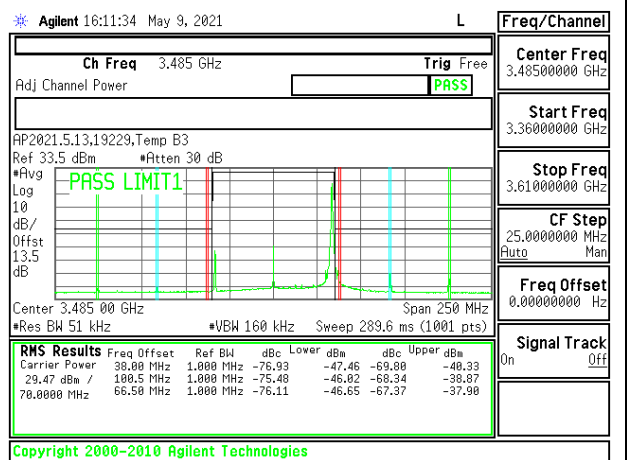
5G NR n77 70MHz BPSK Low Channel RB1-187
