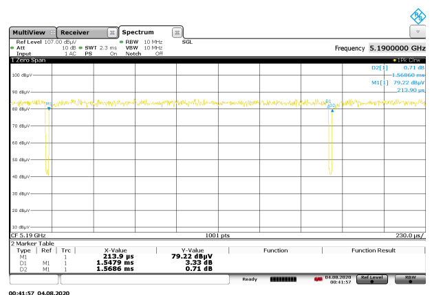
802.11ax HE40 1Tx, MCS11
