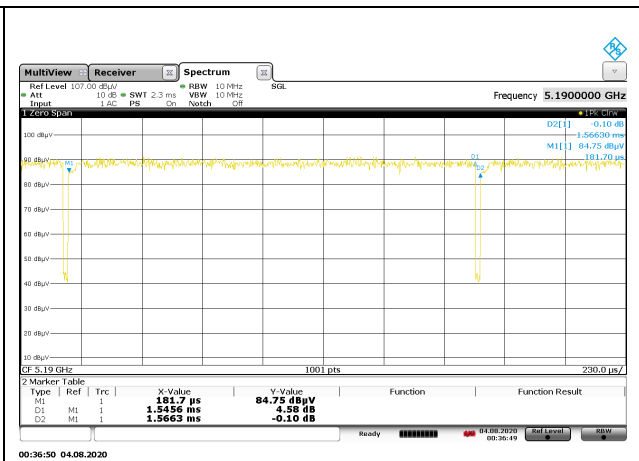
802.11ax HE40 OFDMA, MCS11
