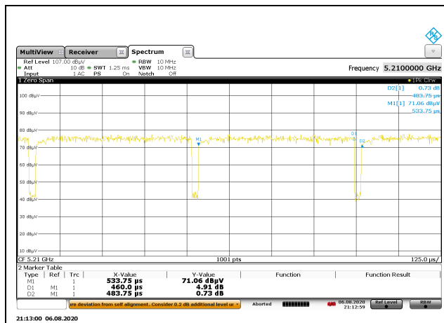
DUTY CYCLE 802.11ac VHT80 1TX MODE MCS0
