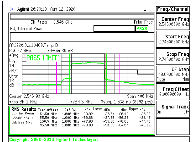
5G NR Band n41 100MHz QPSK Low Channel RB270-0
