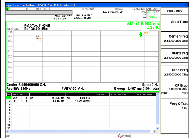
BLE 2Mbps
