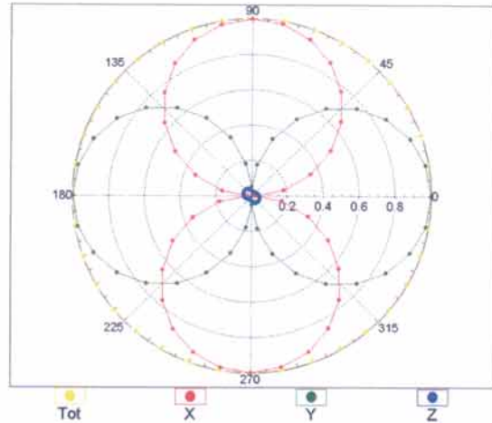
f=2500 MHz, R22, 0^\circ
