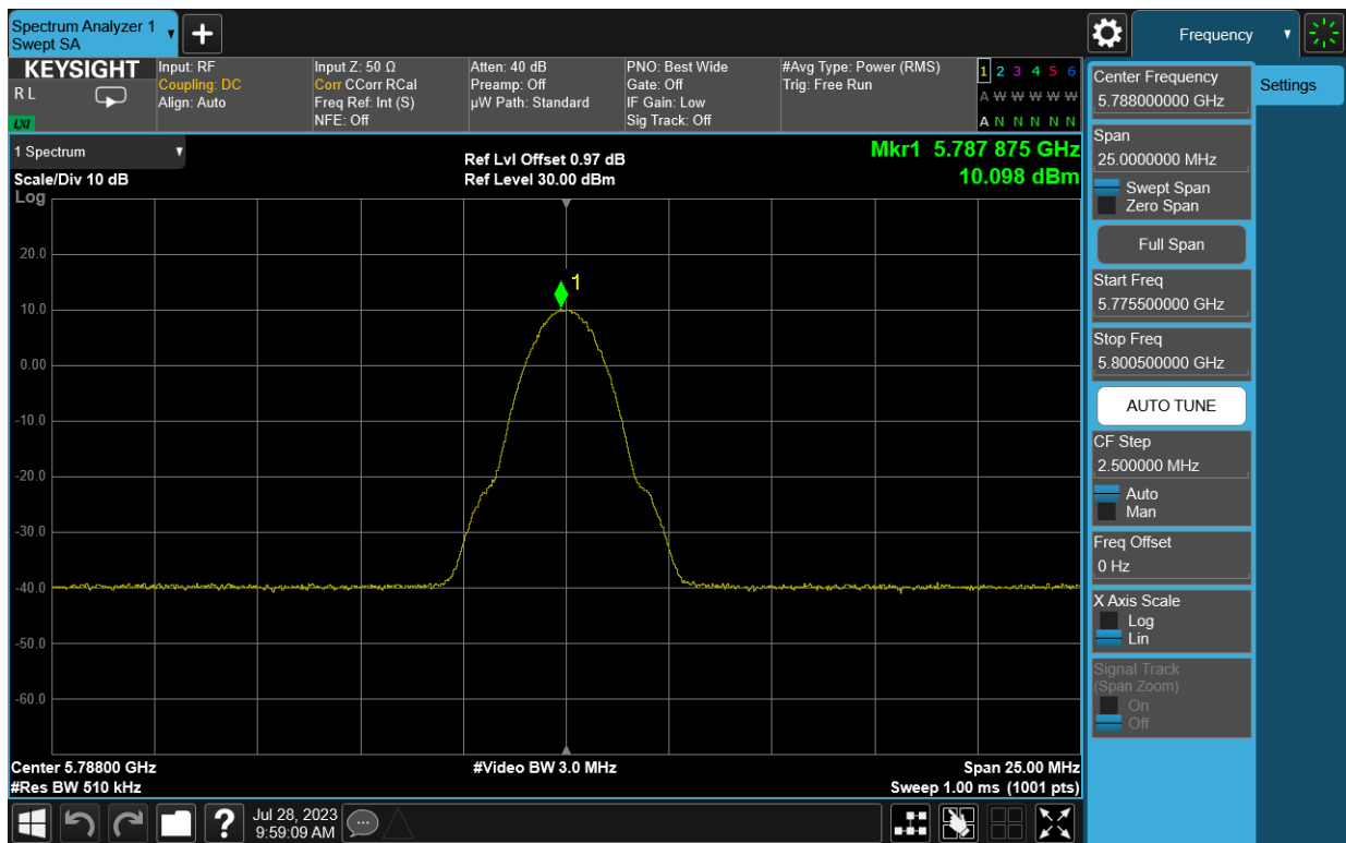
Plot 7-11. PSD (LE2M, 5788MHz)
