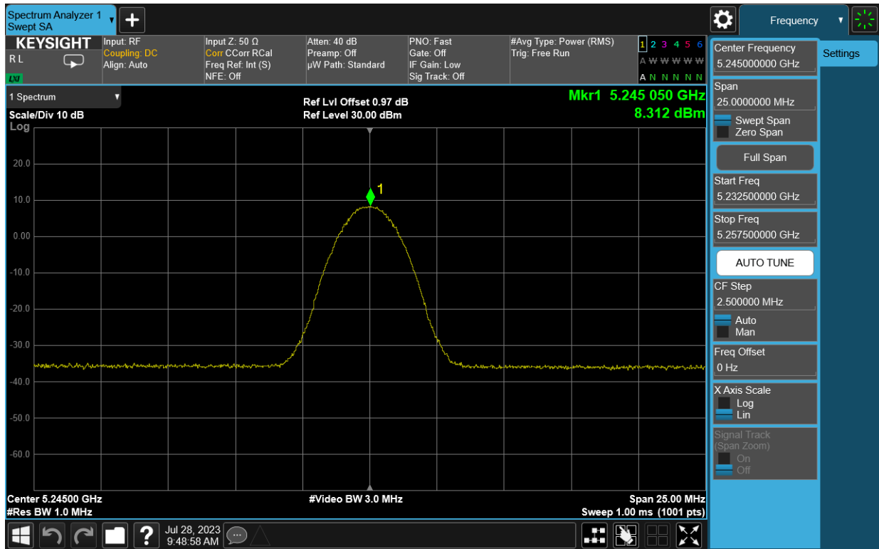
Plot 7-9. PSD (LE2M, 5245MHz)
