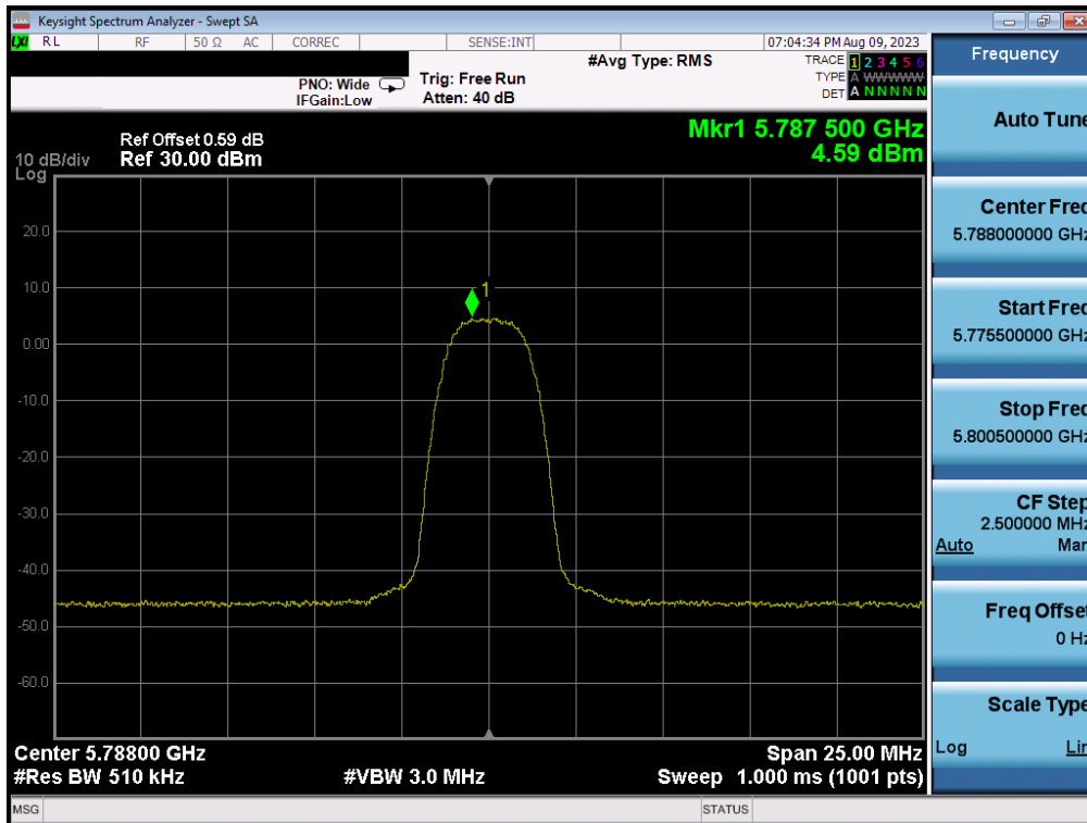
Plot 7-44. PSD (HDRp4 – 5788MHz)
