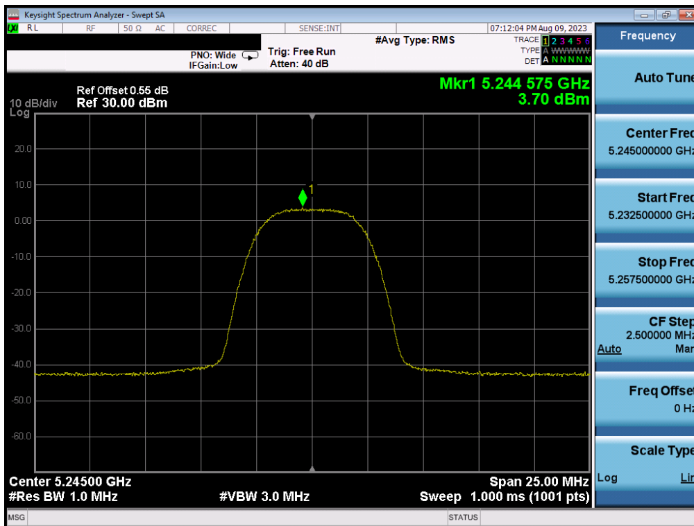
Plot 7-36. (HDRp8 – 5245MHz)
