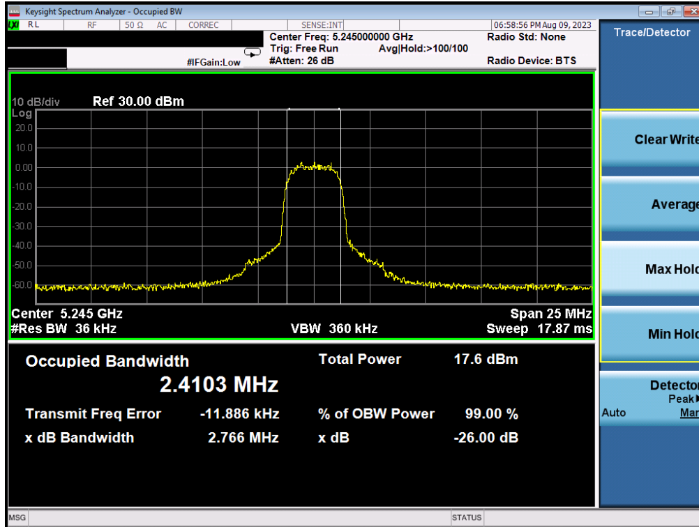
Plot 7-9. 26dB BW & 99% OBW (HDRp4, 5245MHz)
