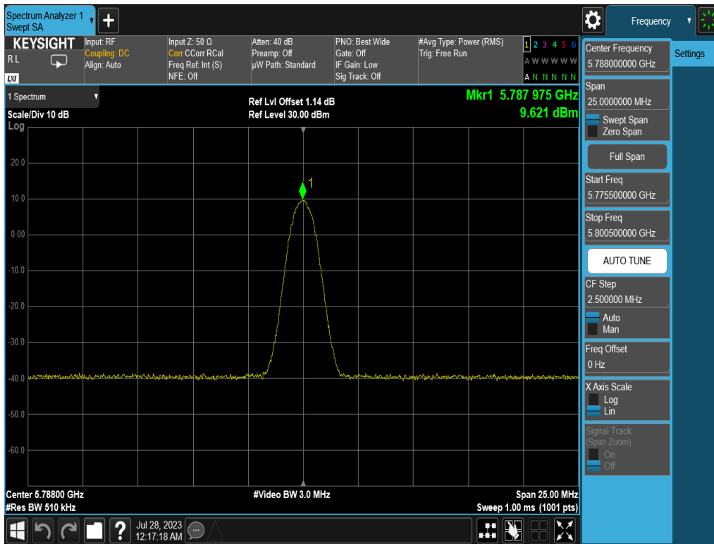
Plot 7-11. PSD (BDR, 5788MHz)
