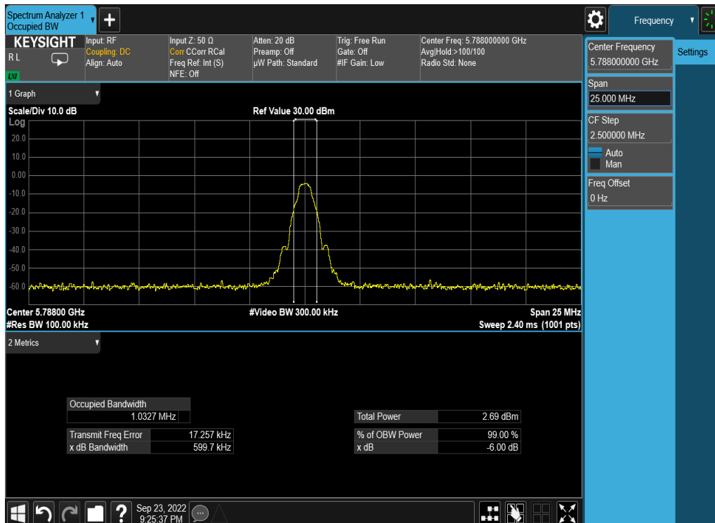
Plot 7-5. 6dB BW & 99% OBW (BDR, 5788MHz)
