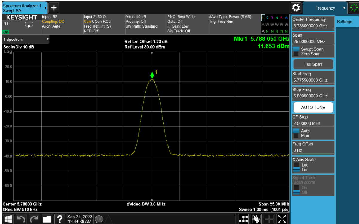
Plot 7-11. PSD (BDR GFSK – 5788MHz)
