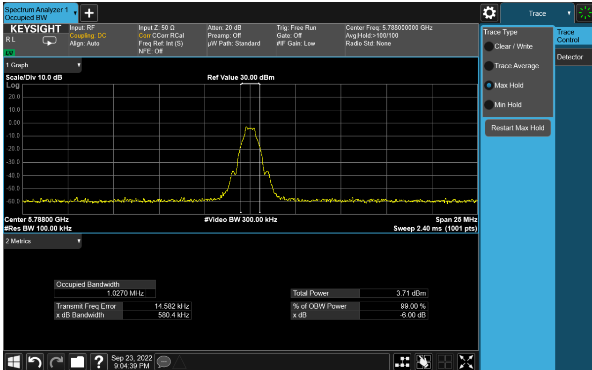
Plot 7-5. 6dB BW & 99% OBW (BDR GFSK – 5788MHz)
