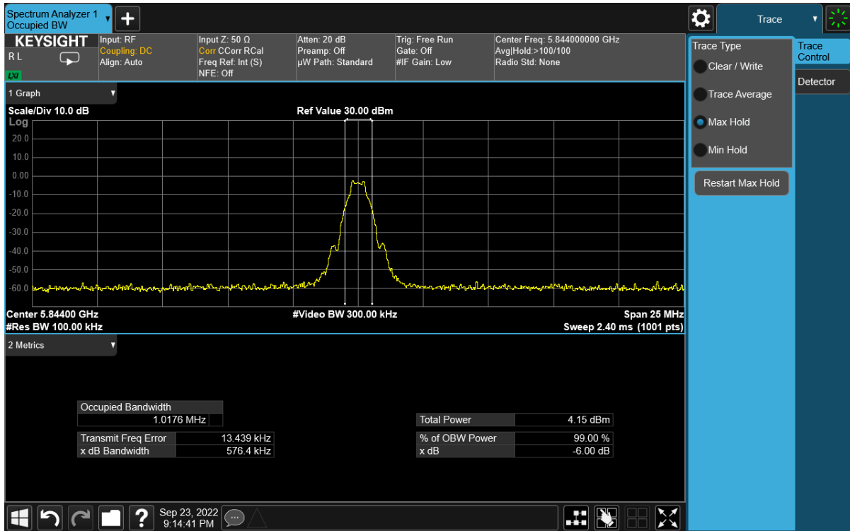
Plot 7-6. 6dB BW & 99% OBW (BDR GFSK – 5844MHz)
