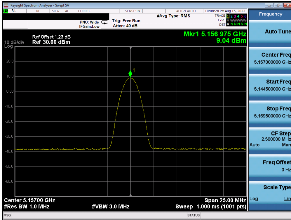
Plot 7-7. PSD (BDR GFSK – 5157MHz)
