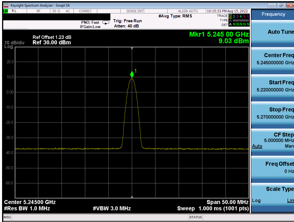
Plot 7-9. PSD (BDR GFSK – 5245MHz)
