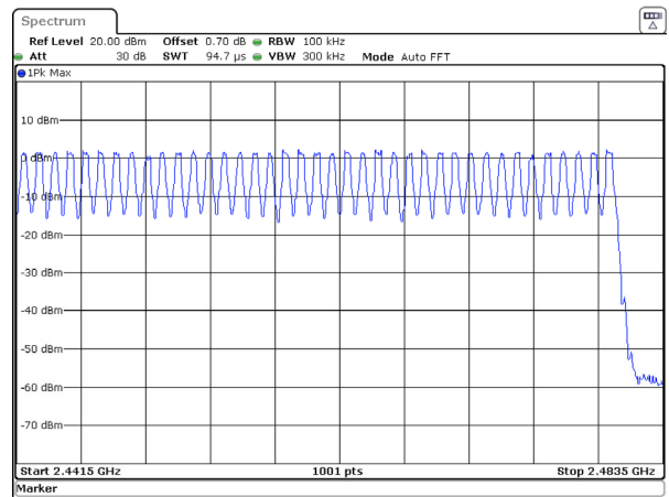
2480 MHz
