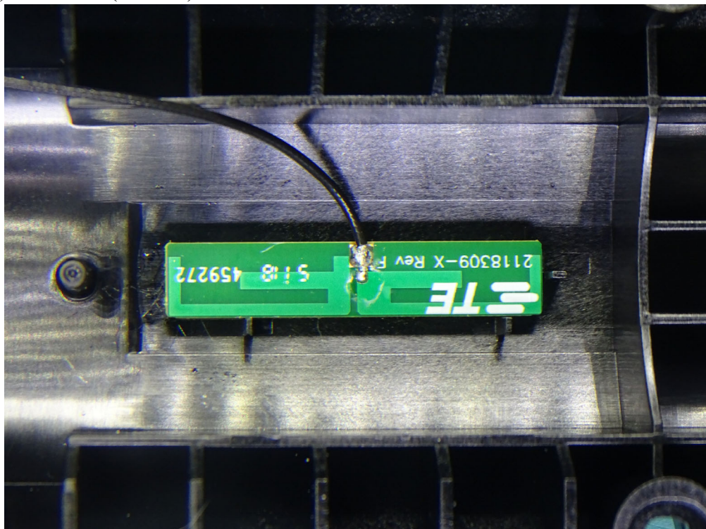
(15) EUT Photo(Antenna)
