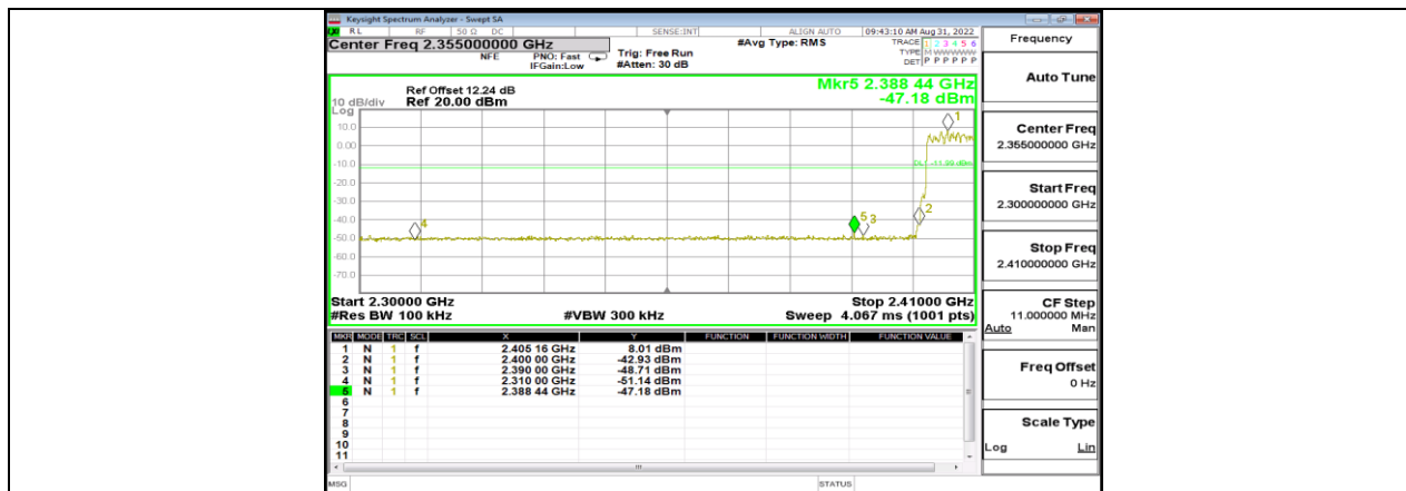
3DH5_Ant1_Low_Hop_2402
