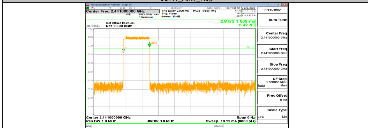
3DH3_Ant1_Hop
