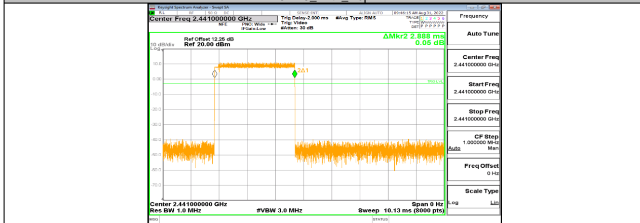
3DH5_Ant1_Hop
