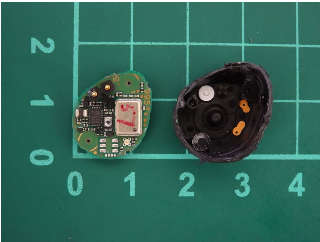
(64) EUT Photo
