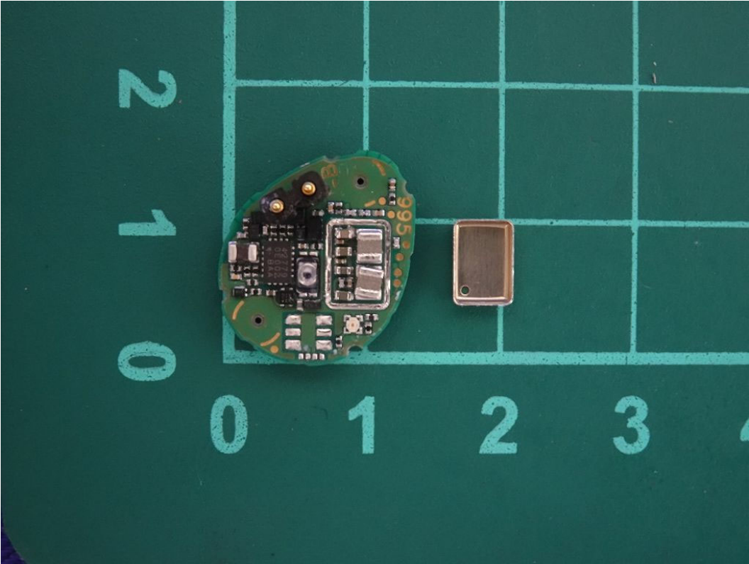
(66) EUT Photo
