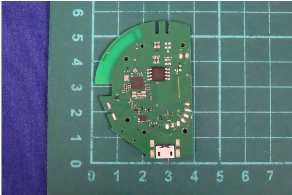
(49) EUT Photo
