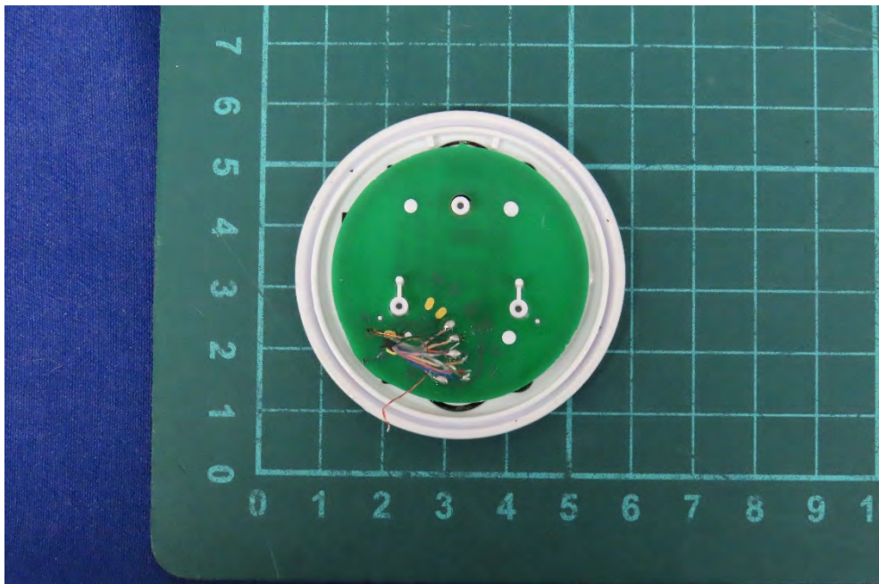
(54) EUT Photo
