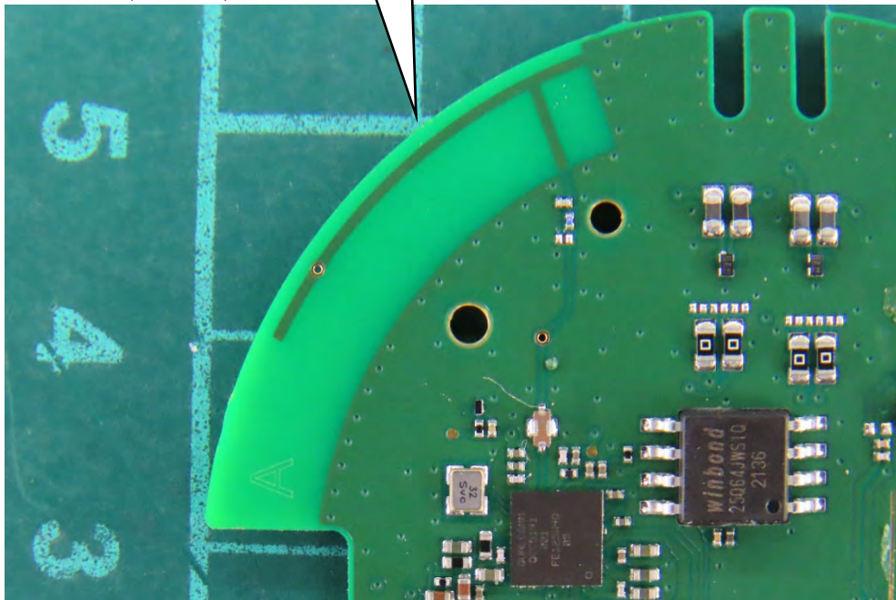
(30) EUT Photo(Antenna)
