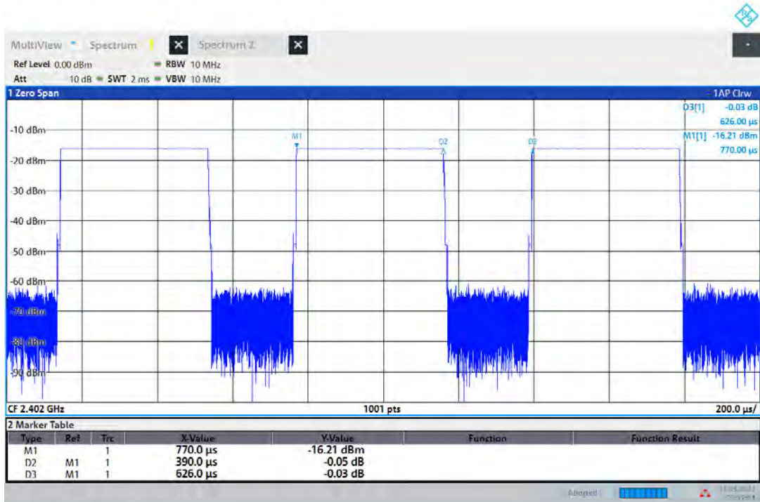
BLE 1M
