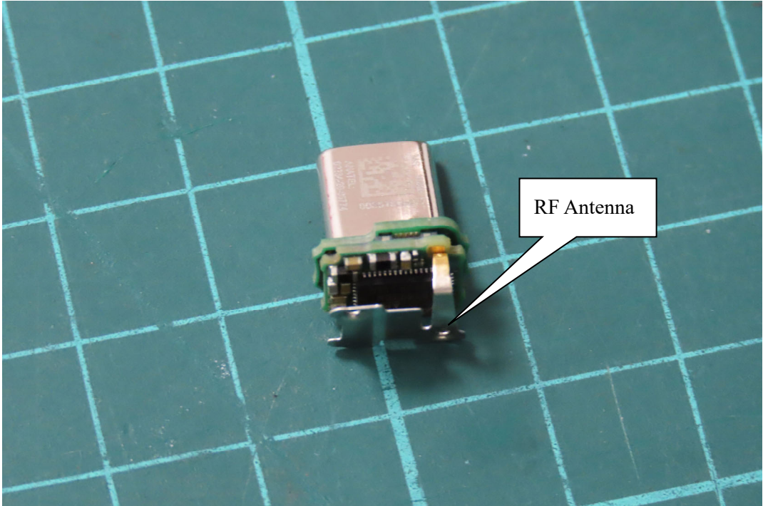
(8) EUT Photo
