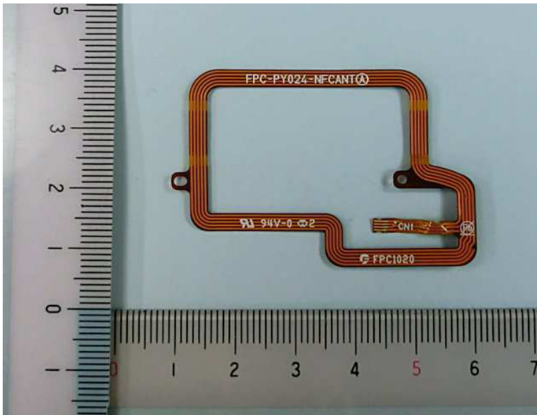
NFC Antenna
