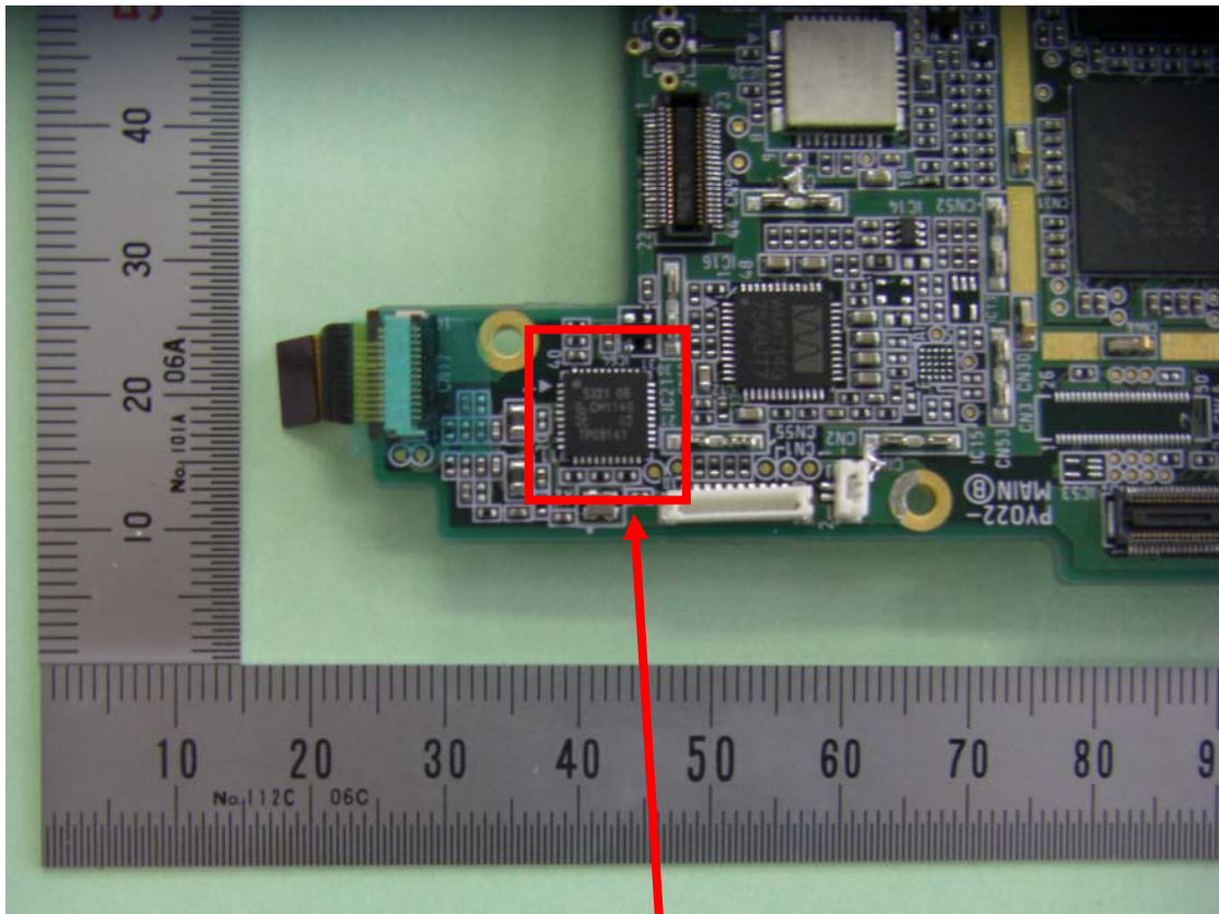
RFID Chip
