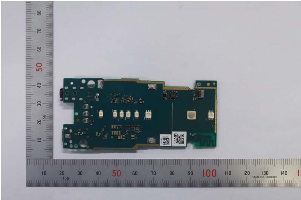
MAIN_bottom
