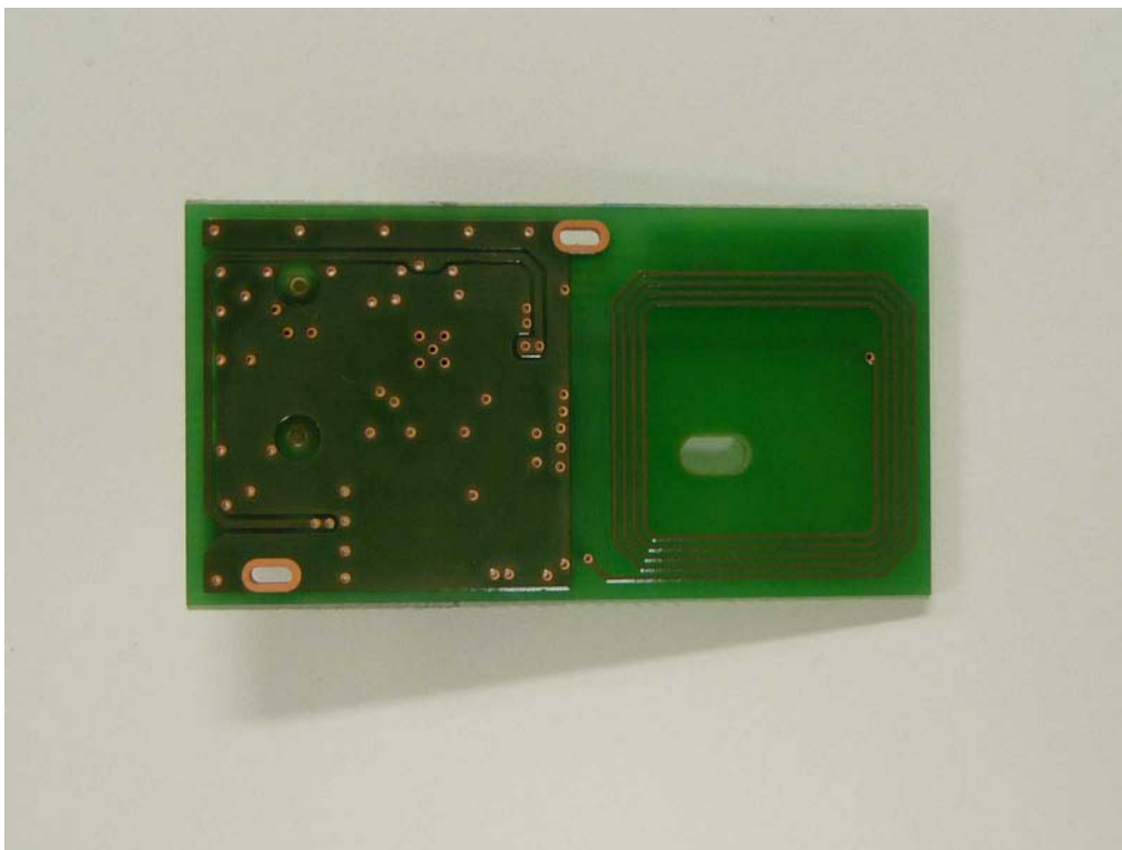
Bottom – 2ch(C)
