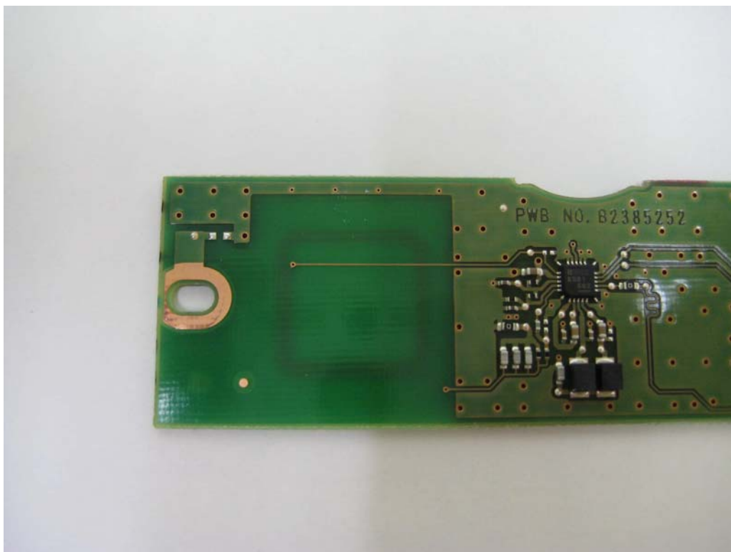
RFID Module Front (Enlarged) - Left
