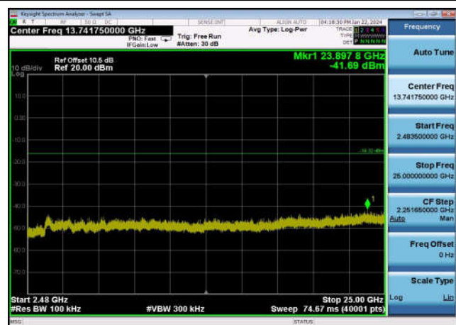
,Plot 4,2483.5MHz~25000MHz-802.11n(HT20),2462MHz,Ant0
