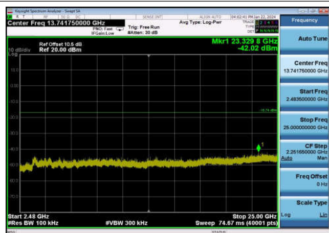
,Plot 4,2483.5MHz~25000MHz-802.11n(HT20),2462MHz,Ant0
