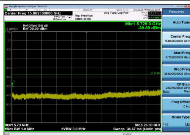
U-NII-2c ,Plot 3,5725MHz~26000MHz-802 .11ac(40MHz),5510MHz,Ant1
