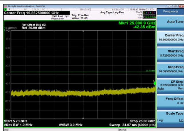
U-NII-2c ,Plot 3,5725MHz~26000MHz-802 .11ac(80MHz),5530MHz,Ant1
