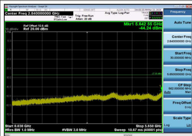
U-NII-3 ,Plot 2,30MHz~5650MHz-802.11a (20MHz),5825MHz,Ant1
