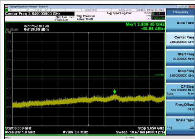
U-NII-3 ,Plot 2,30MHz~5650MHz-802.11a c(20MHz),5785MHz,Ant1
