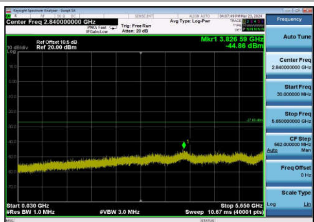
U-NII-3 ,Plot 2,30MHz~5650MHz-802.11a c(20MHz),5745MHz,Ant1
