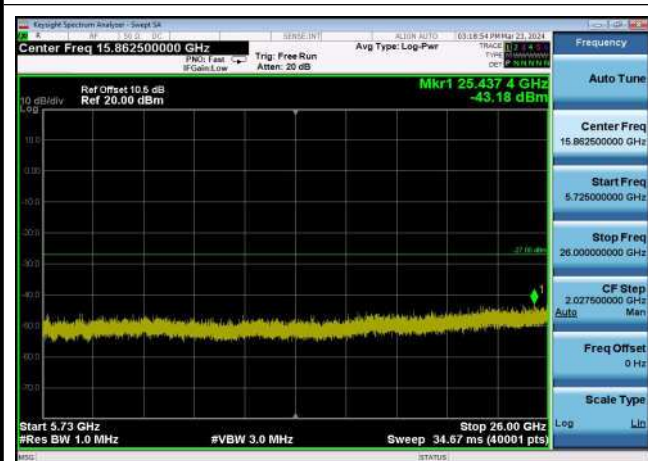
U-NII-2c ,Plot 3,5725MHz~26000MHz-802 .11n(20MHz),5700MHz,Ant1
