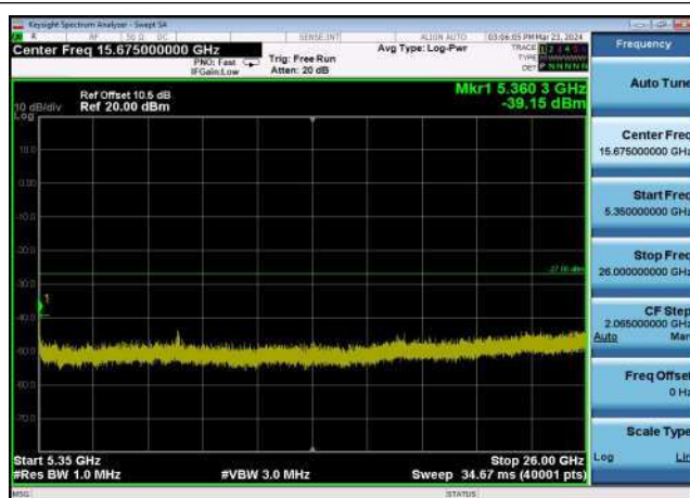
U-NII-2a ,Plot 3,5350MHz~26000MHz-802 .11ac(40MHz),5270MHz,Ant1
