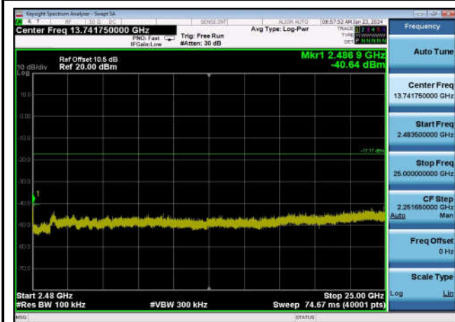
,Plot 4,2483.5MHz~25000MHz-802.11n(HT40),2437MHz,Ant0
