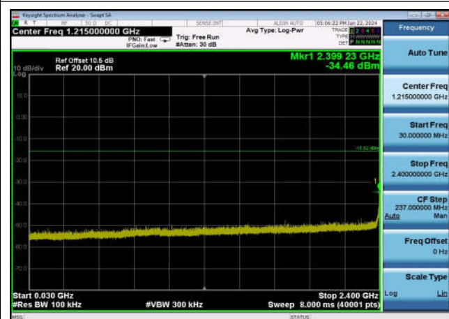
,Plot 3,30MHz~2400MHz-802.11g,2462MHz
