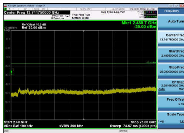
,Plot 4,2483.5MHz~25000MHz-802.11n(HT40),2452MHz,Ant0
