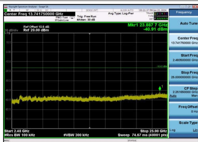
,Plot 4,2483.5MHz~25000MHz-802.11n(HT20),2462MHz,Ant0
