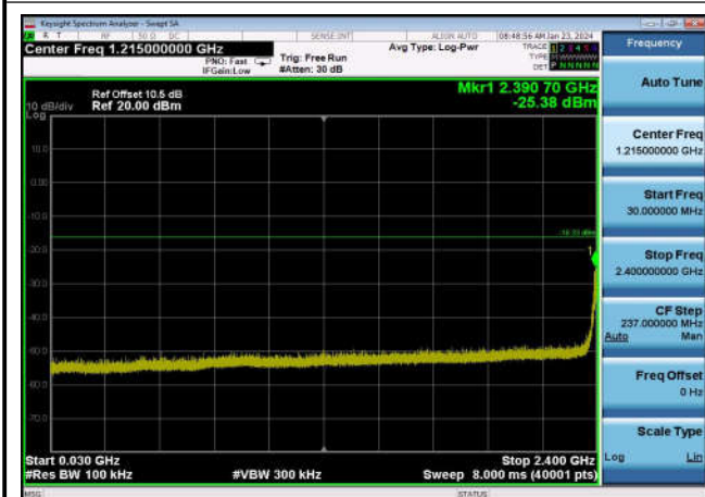
,Plot 3,30MHz~2400MHz-802.11n(HT40) ,2452MHz,Ant0
