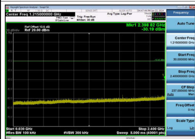
,Plot 3,30MHz~2400MHz-802.11b,2462MHz
