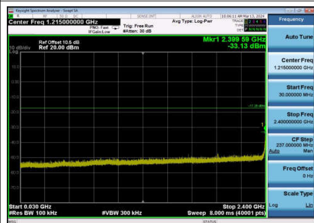
,Plot 3,30MHz~2400MHz-802.11n(20MHz) ,2462MHz,Ant0
