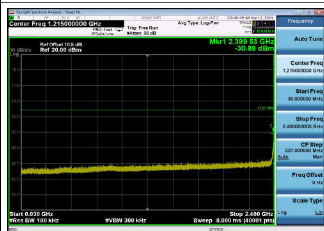
,Plot 3,30MHz~2400MHz-802.11g,2462MHz
