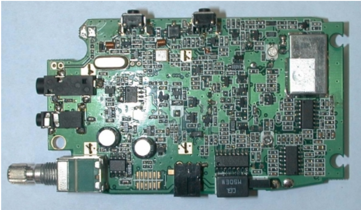
PCB Bottom
