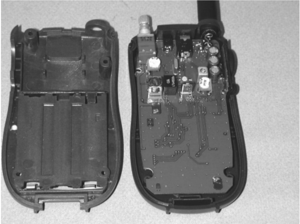
PCB Bottom
