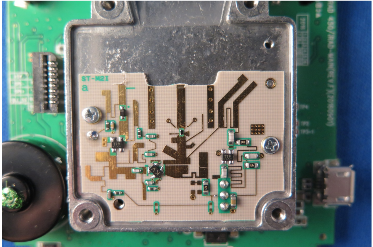
LNA PCB
