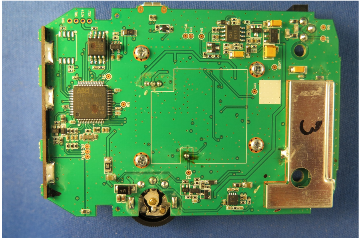
BOTTOM PCB
