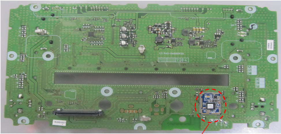
Bluetooth Module
