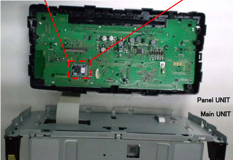
Bluetooth MODULE
