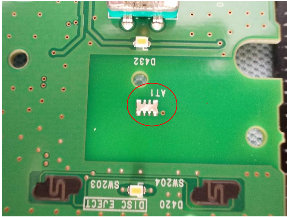
Antenna
