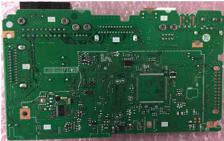
【AUDIO_PCB(Solder side)】
