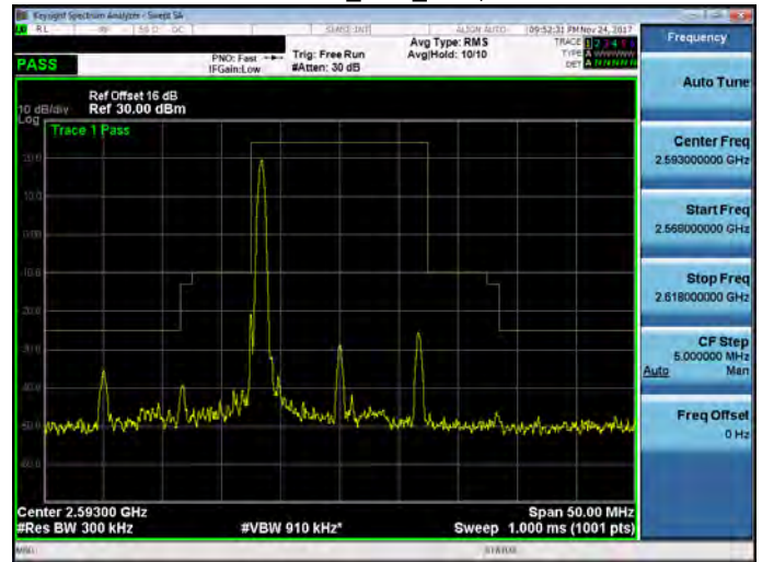
Band 41_15M_RB1,74
