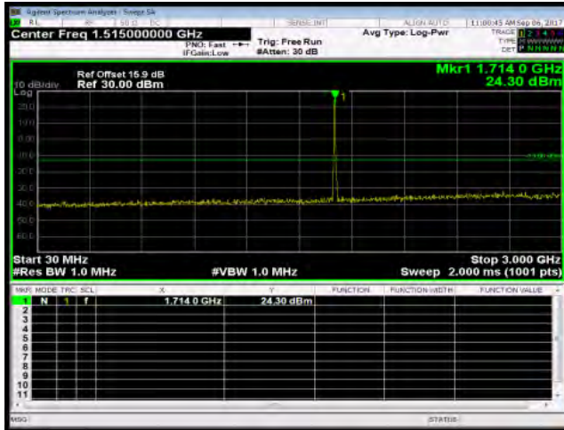
30MHz~3GHz_WCDMA_B4_LowCH1312-1712.4
