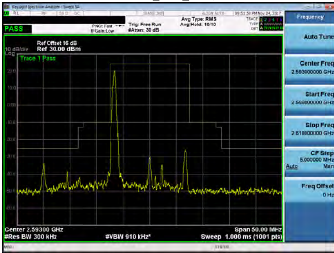
Band 41_15M_RB1,74
