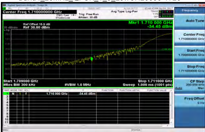
Band4_20MHz_QPSK_1_0_LowCH20050-1720
