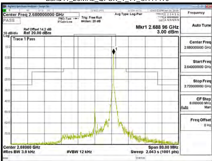
Band41_20MHz_QPSK_1_99_CH41490
