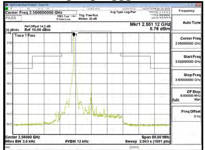
Band7_20MHz_QPSK_1_0_CH21350
