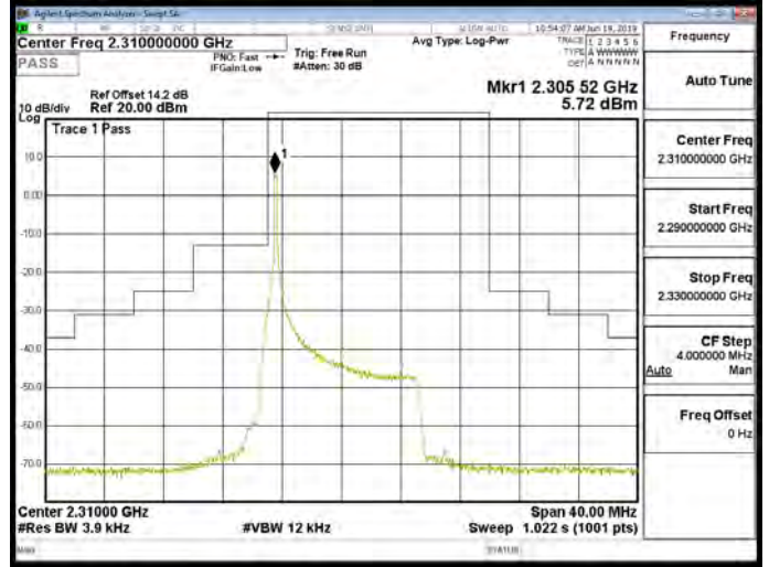
Band30_10MHz_QPSK_1_49_CH27710
