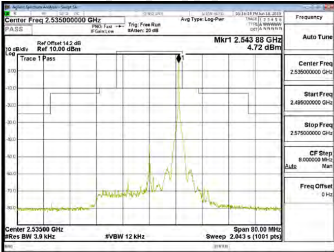
Band7_20MHz_QPSK_1_99_CH21350
