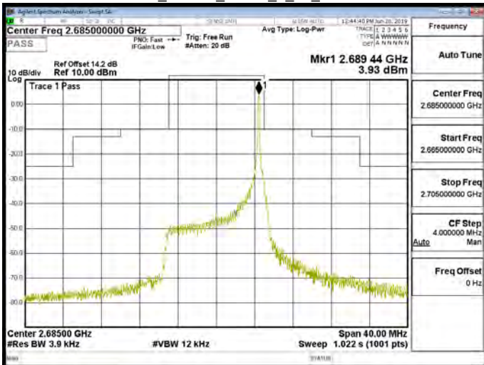
Band41_10MHz_QPSK_1_49_CH41540
