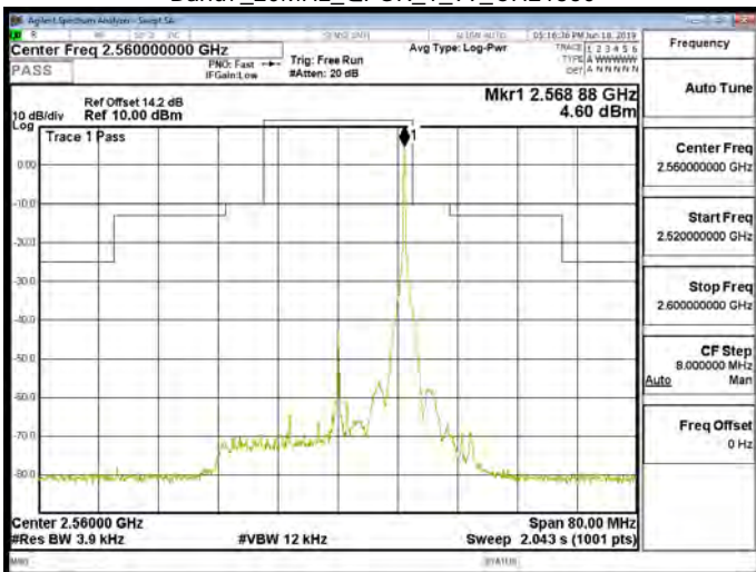
Band7_20MHz_QPSK_1_99_CH21350
