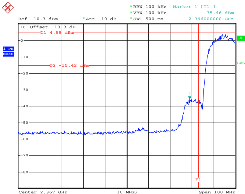
802.11b CH01
