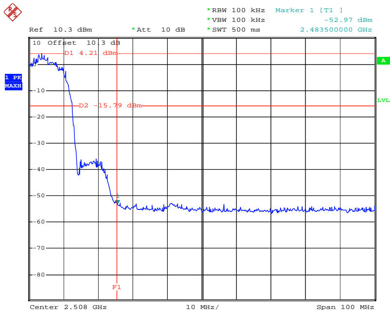
802.11b CH11
