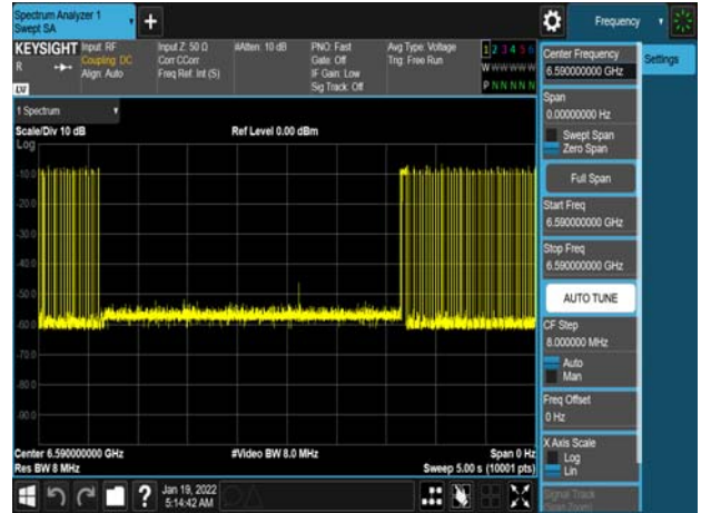
Det Le1_802.11ax_160MHz_6590MHz_-66dBm
