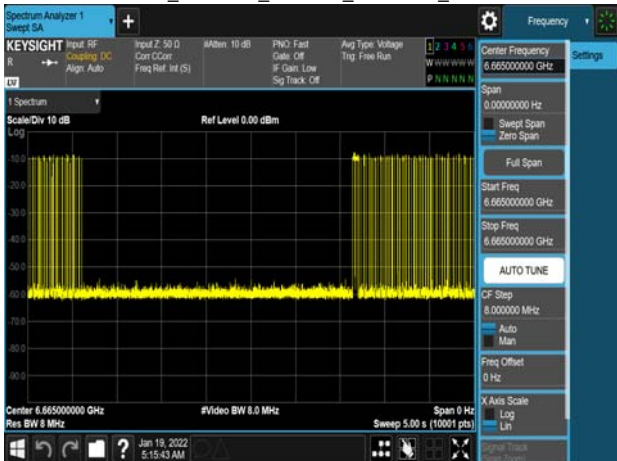
Det Le1_802.11ax_160MHz_6665MHz_-64dBm
