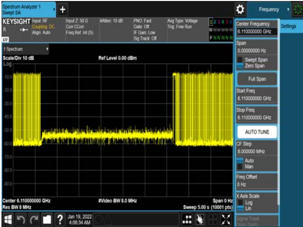
Det LeI_802.11ax_160MHz_6110MHz_-67dBm
