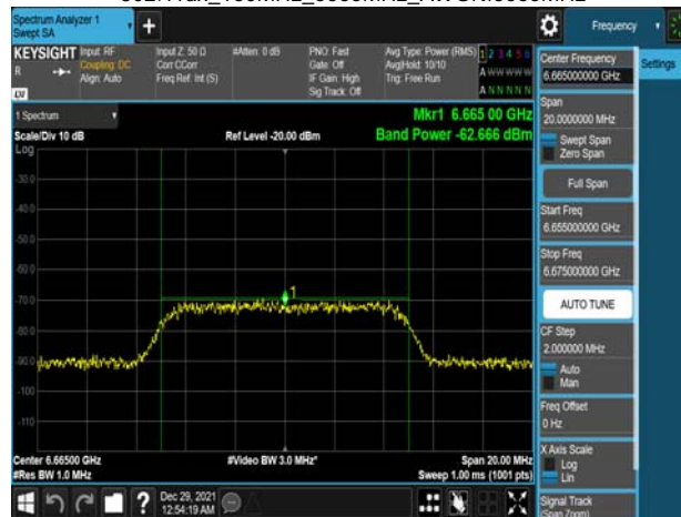
802.11ax_160MHz_6665MHz_AWGN:6665MHz
