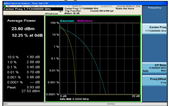
HSUPA_B4_LowCH1312-1712.4
