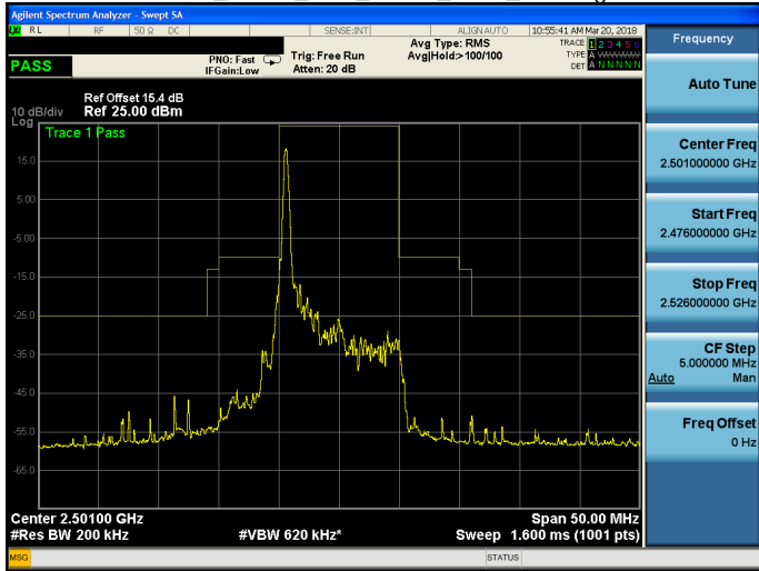
Band 41_QPSK_10M_QPSK_LOW_RB1,49.gif
