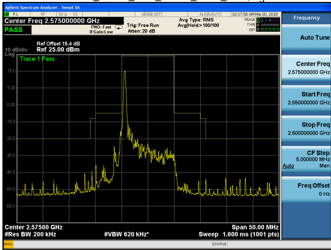
Band 38_QPSK_10M_QPSK_LOW_RB1,49.gif
