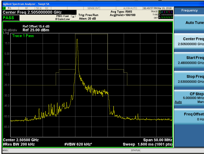
Band 7_QPSK_10M_QPSK_LOW_RB1,49.gif
