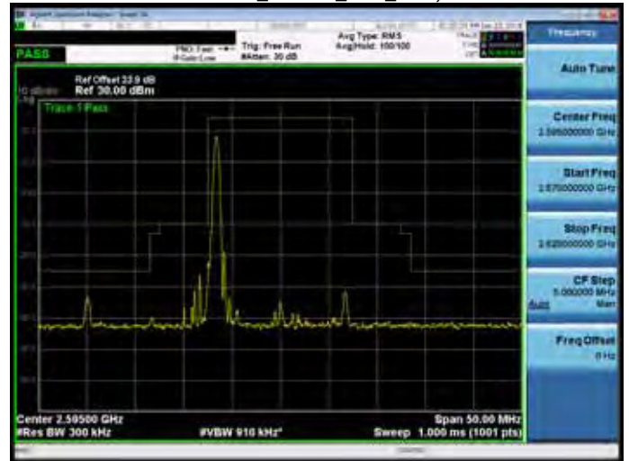
Band 38_16QAM_15M_RB1,74
