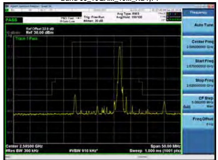
Band 38_16QAM_15M_RB1,74
