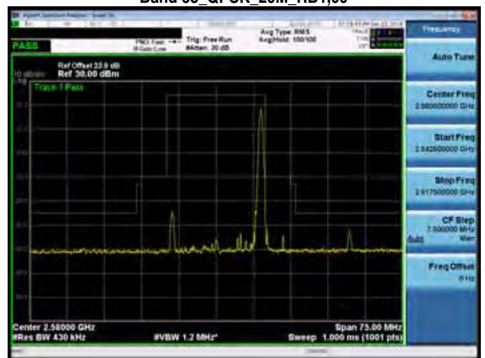
Band 38_QPSK_20M_RB1,99
