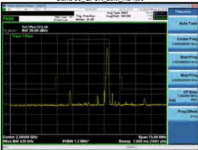
Band 38_QPSK_20M_RB1,99
