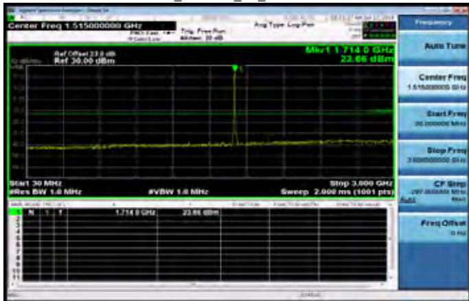
30MHz~3GHz_WCDMA_B4_LowCH1312-1712.4
