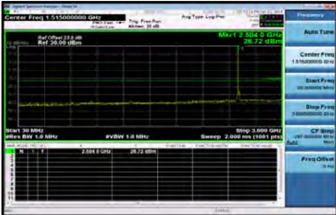
30MHz-3GHz_Band7_20MHz_QPSK_1_0_LowCH20850-2510
