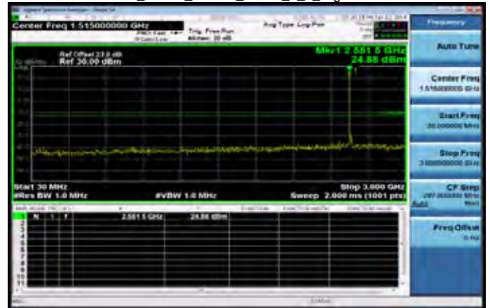
30MHz-3GHz_Band7_20MHz_QPSK_1_0_HighCH21350-2560
