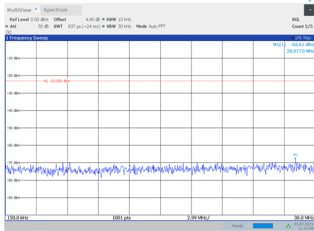
Band4-20MHz-QPSK-19975-1RB#0-Range2:0.15~30MHz
