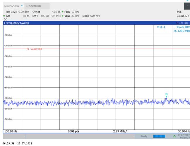
Band26-5MHz-QPSK-26715-1RB#0-Range2:0.15~30MHz
