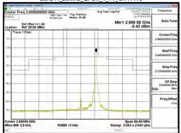
Band41_20MHz_QPSK_1_99_CH41490
