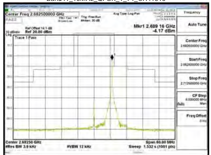
Band41_15MHz_QPSK_1_74_CH41515
