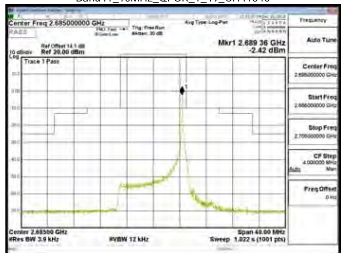
Band41_10MHz_QPSK_1_49_CH41540
