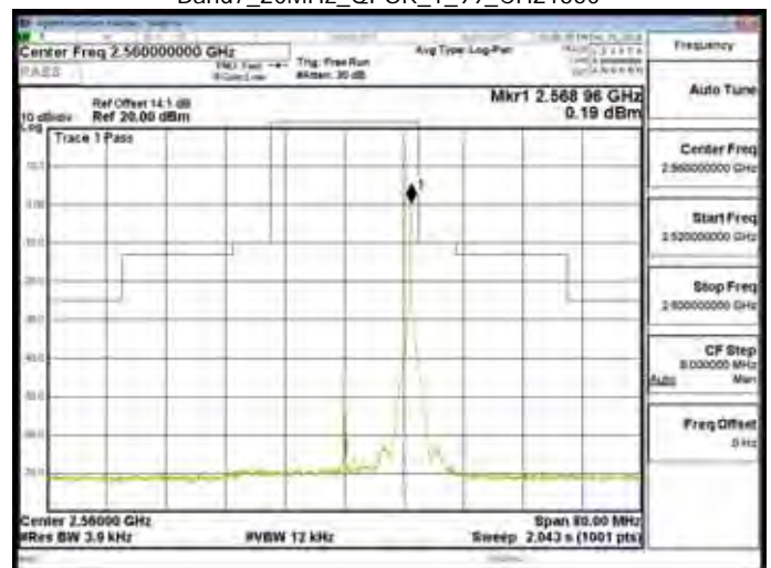
Band7_20MHz_QPSK_1_99_CH21350
