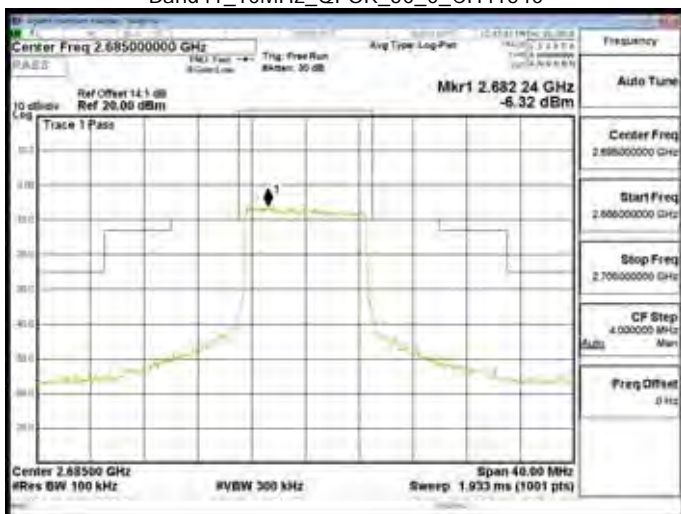
Band41_10MHz_QPSK_50_0_CH41540
